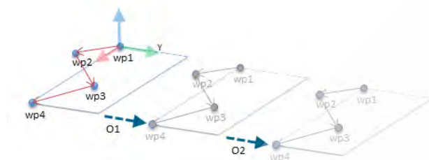
13.6: Stosowanie przesunięcia do funkcji płaszczyzny
